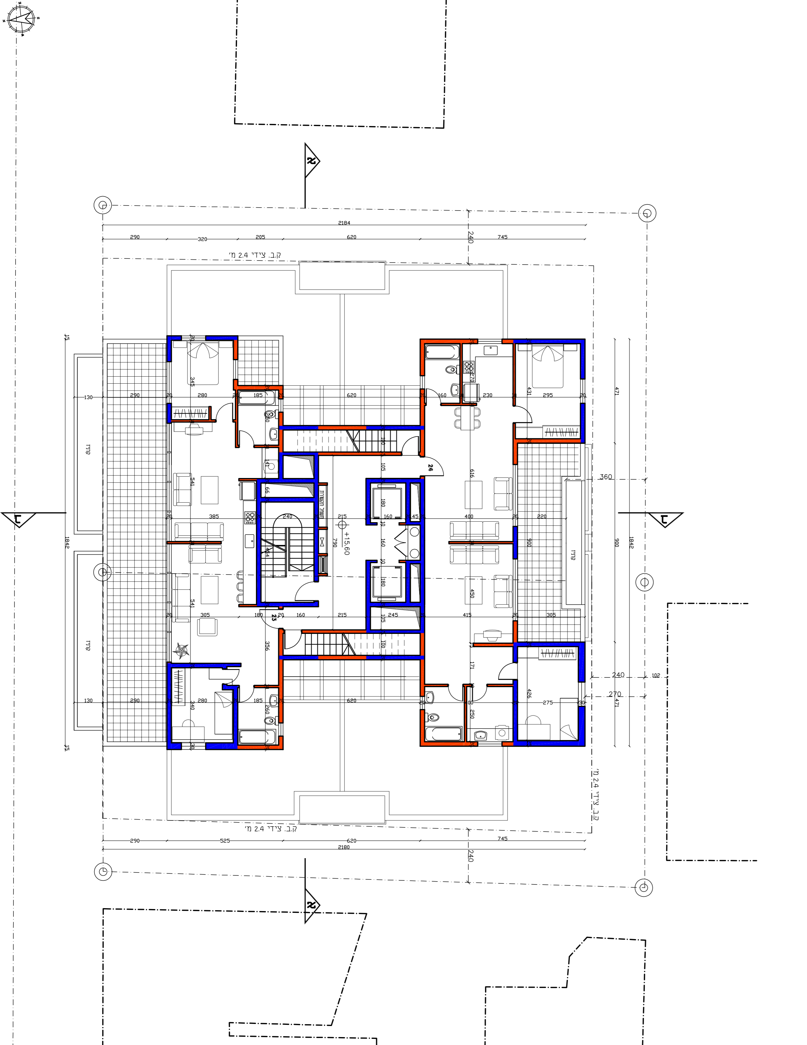
תוכנית קומה 3 - חלק א' (מבט צפון)
